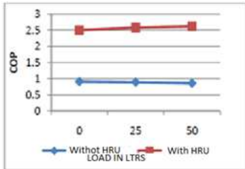
Fig.6 Actual Overall COP Vs.Load
